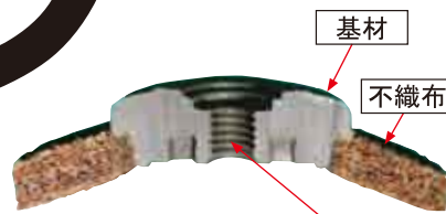
M10 ネジ式でクイック脱着が可能
